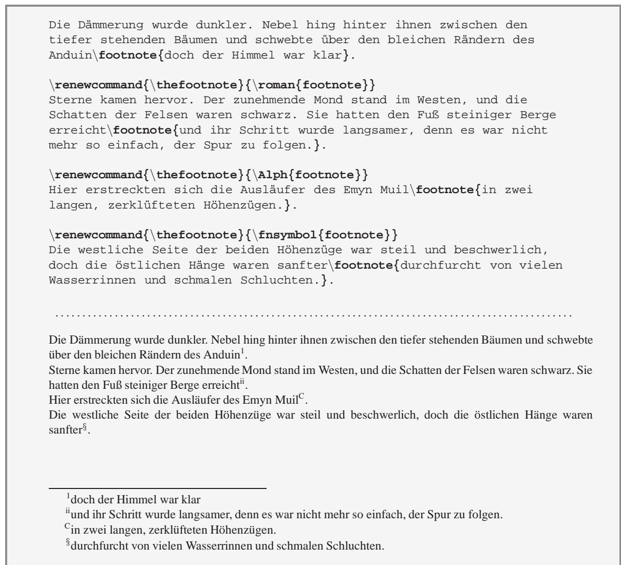
Abbildung 5: Ausgabe von Zählern
