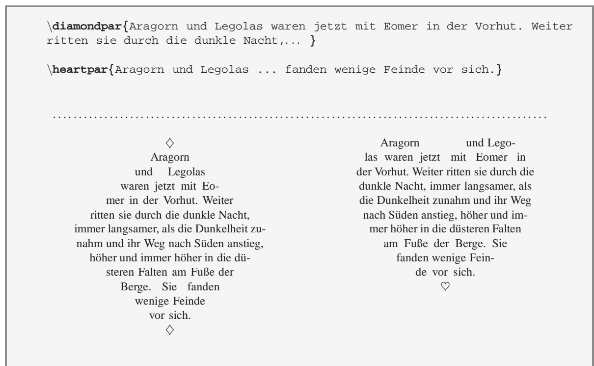
Abbildung 53: Formen von Absätzen mit shapepar
