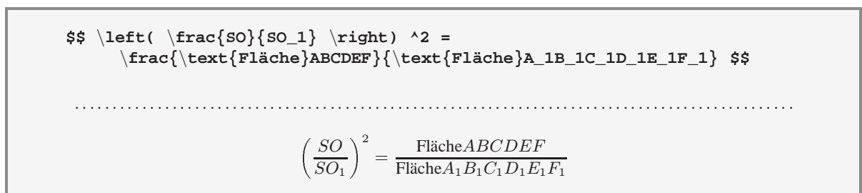
Abbildung 40: Mathematikmodus: Texteingaben
