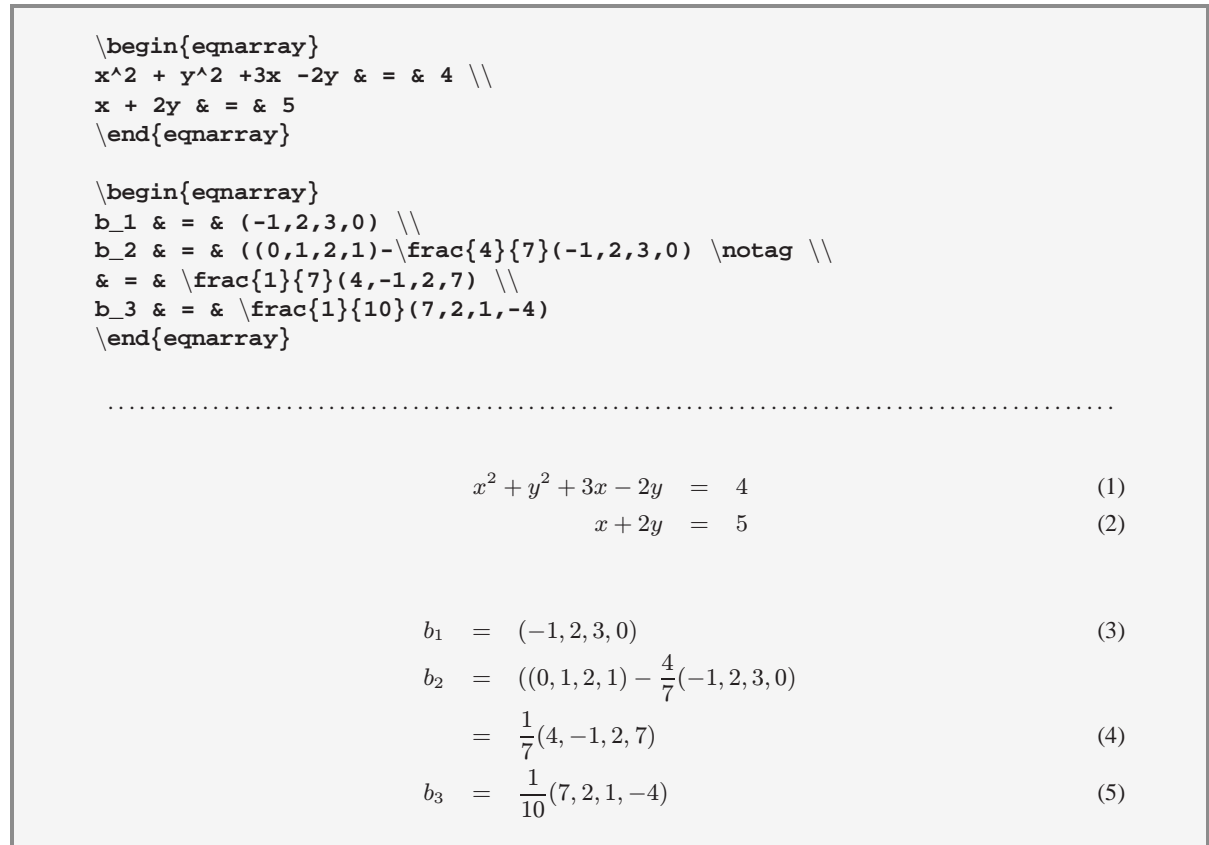
Abbildung 46: Mathematikmodus: Gleichungssysteme
