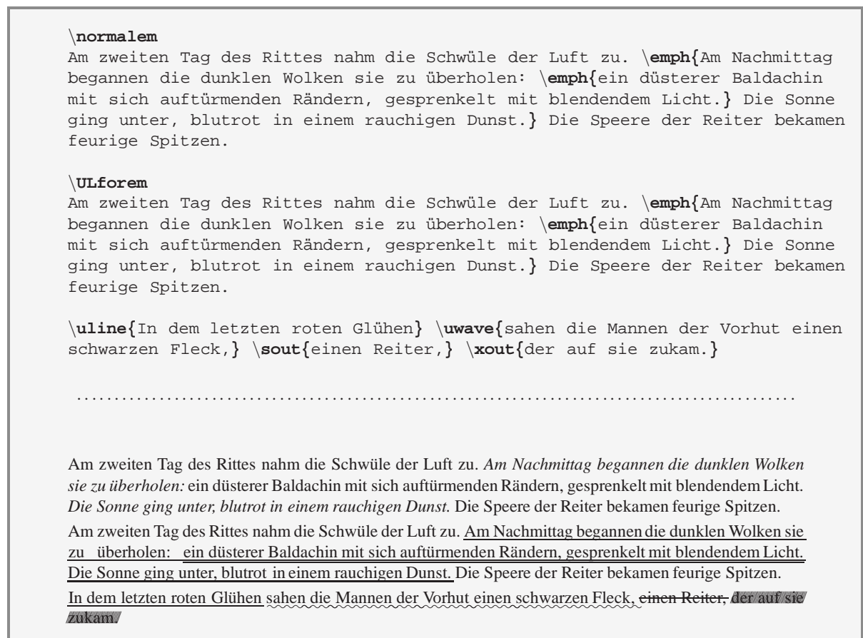
Abbildung 52: Hervorheben von Wörtern mit ulem
