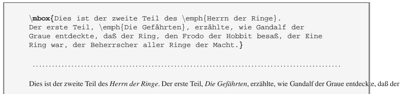
Abbildung 1: Der LR-Modus
