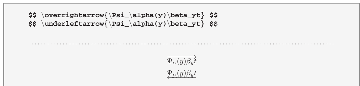
Abbildung 38: Mathematikmodus: Pfeile
